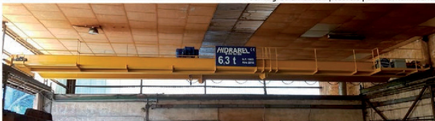
Puente grúa birraíl con pasarela para mantenimiento
